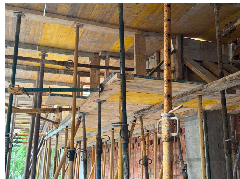
Fotografía 3. Encofrado para forjado cubre-baja
