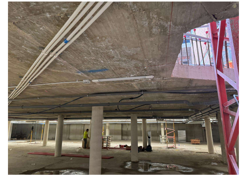
Fotografía 3. Trabajos en planta sótano. Inst iluminación
