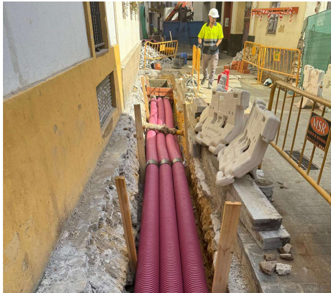
Fotografía 1. Trabajos para acometida de electricidad
