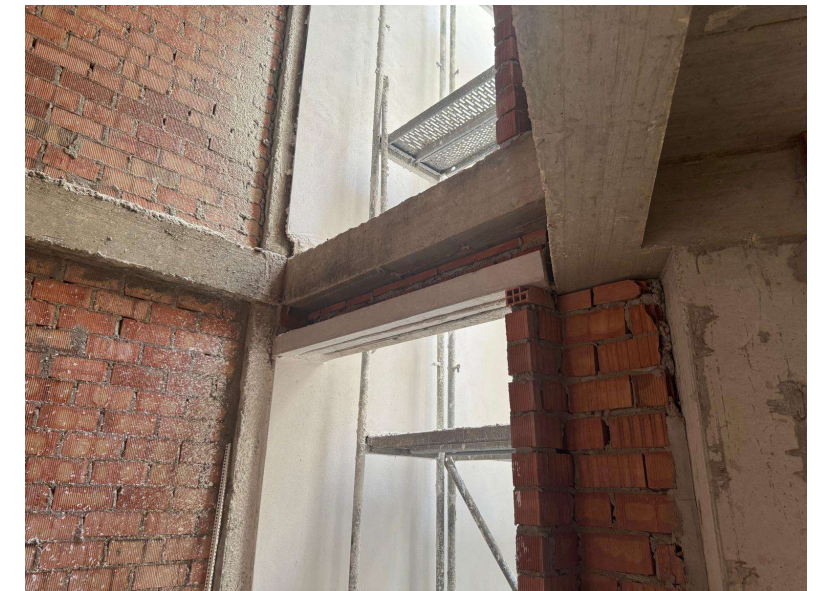
Fotografía 6. Continúan trabajos interiores viviendas taller
