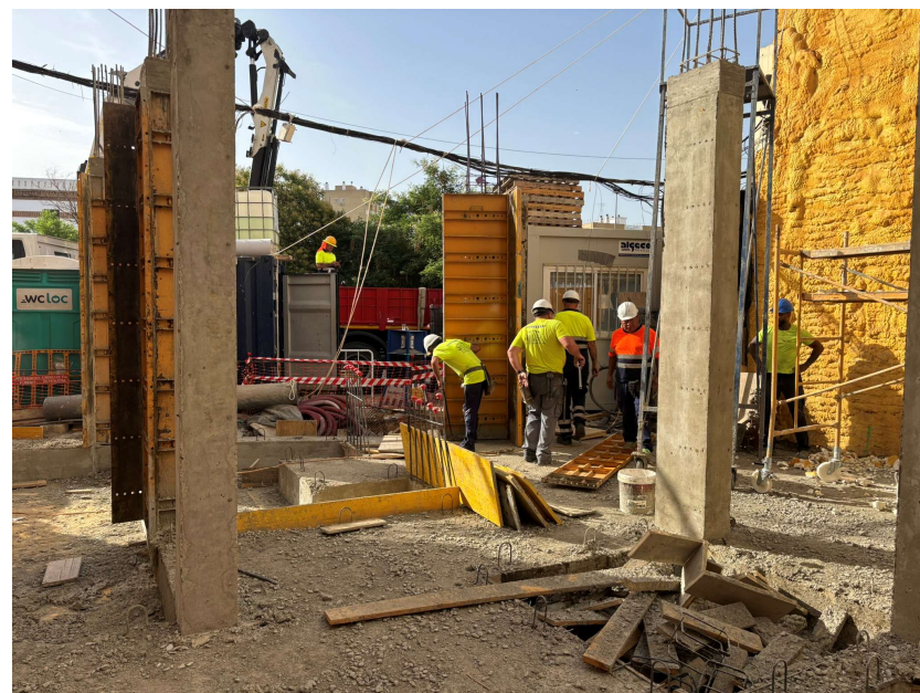
Fotografía 1. Desencofrado de pilares terminados P. Baja
