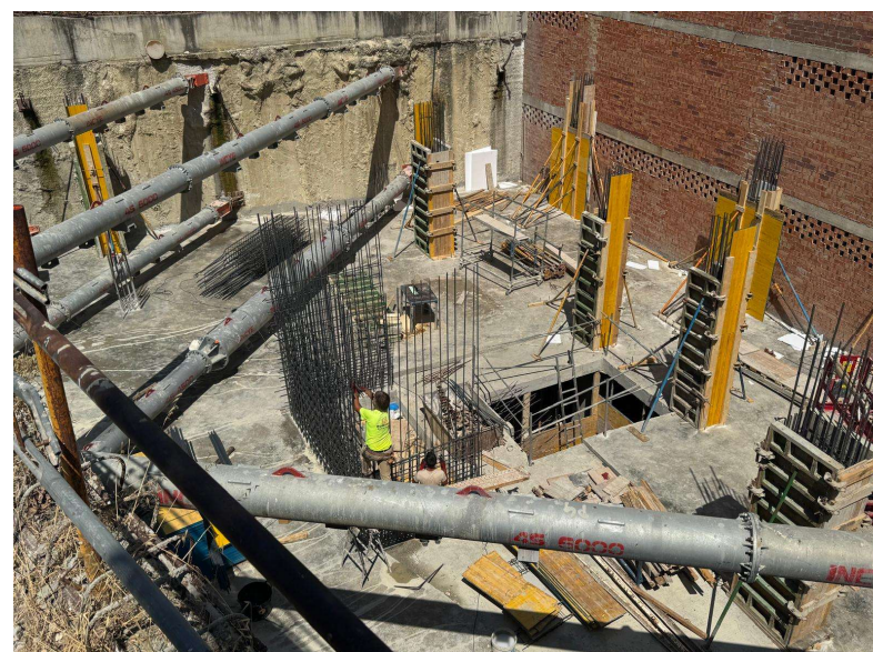
Fotografía 5. Encofrado pilares planta sótano -2
