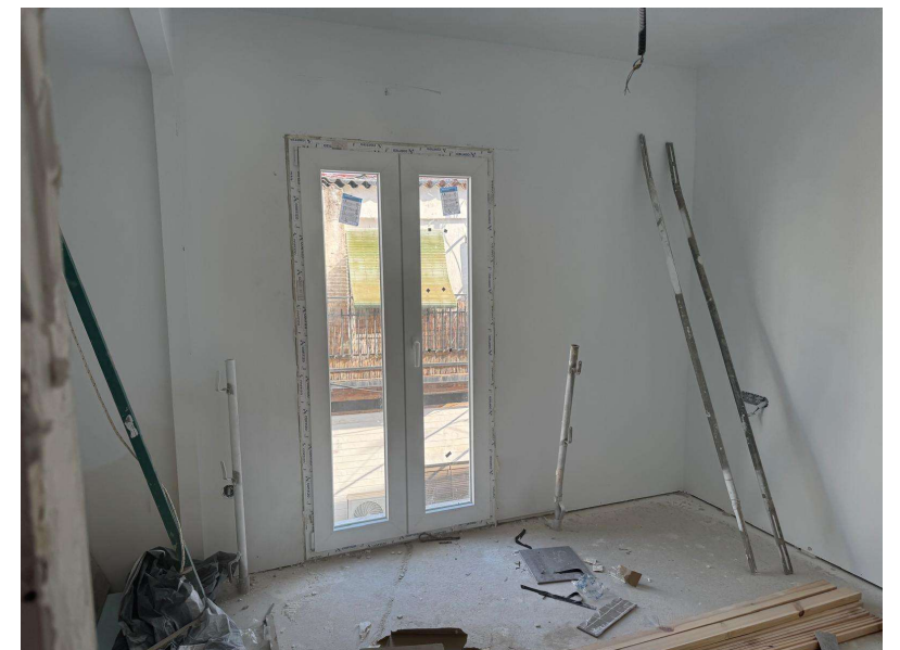
Fotografía 3. Instalación de carpinterías exteriores
