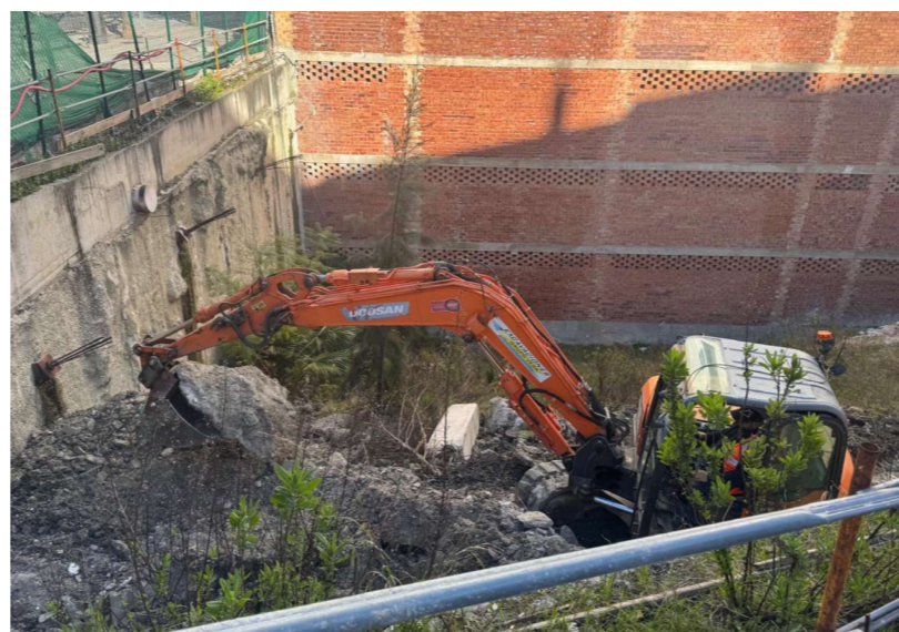
Fotografía 5. Retirada de escombros preexistentes
