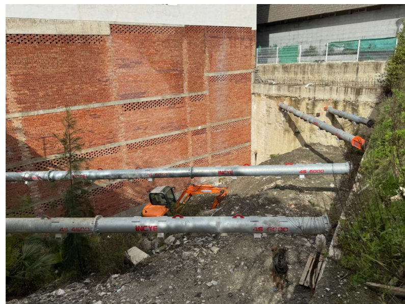
Fotografía 1. Acodamiento de Pantallas
