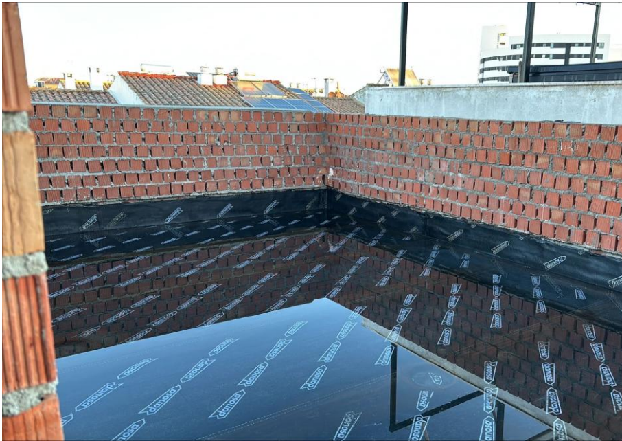
Fotografía 2. Finalización pruebas de estanqueidad en cubiertas.
