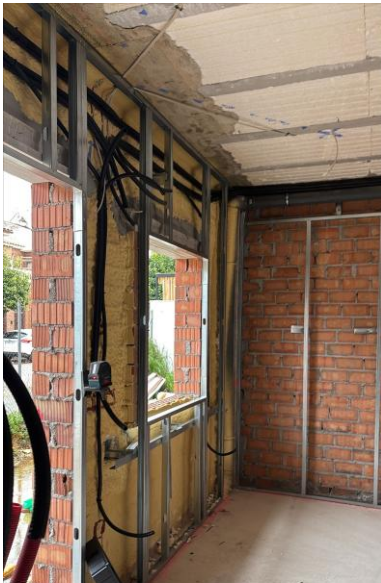
Fotografía 5. Colocación de corrugados para electricidad.
