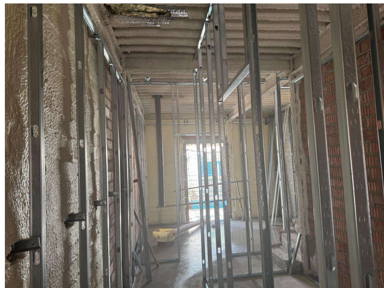
Fotografía 4. Inicio trabajos tabiquería seca
