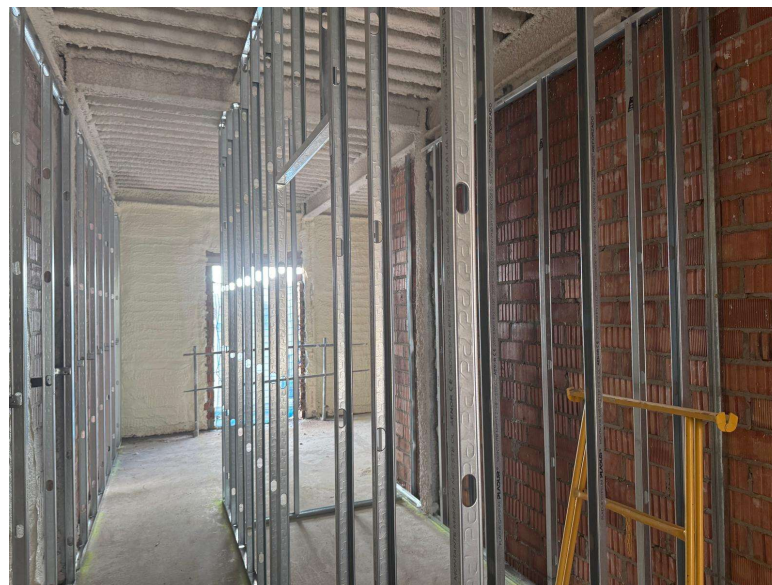
Fotografía 5. Inicio trabajos tabiquería seca
