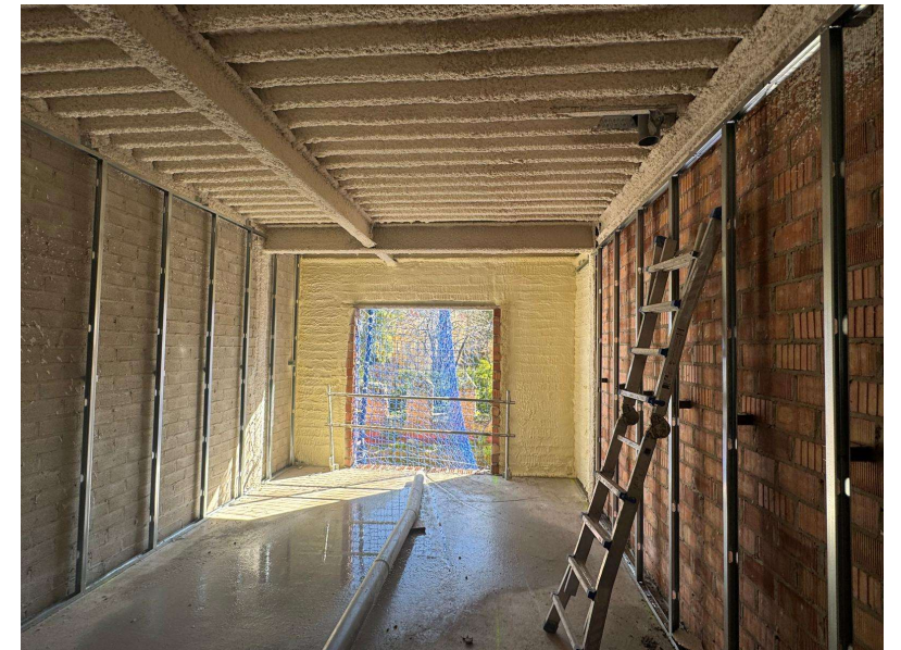
Fotografía 3. Cerramiento con espuma de poliuretano
