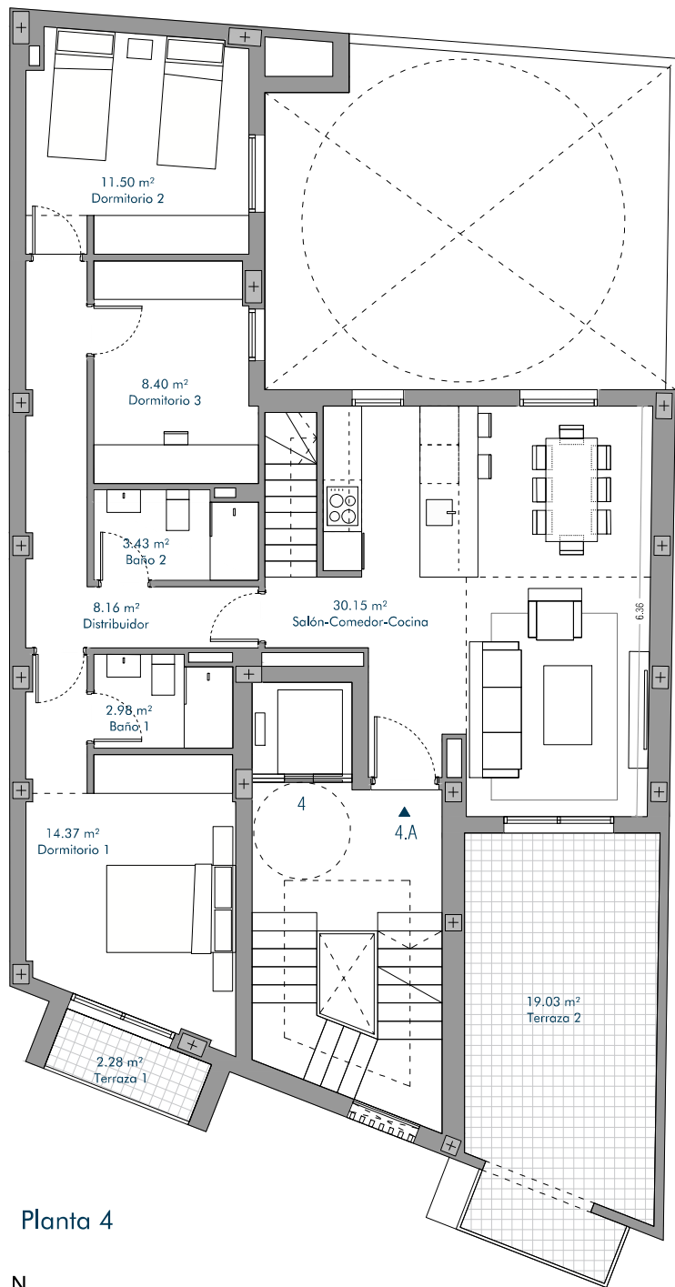
Planta Ático
